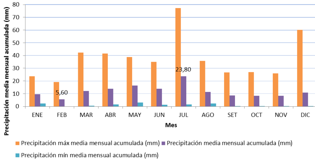
Figura 3-8. Precipitaciones medias, máximas y mínimas medias mensuales acumuladas. Estación Meteorológica Charles Fuhr (período 1955-2014).
