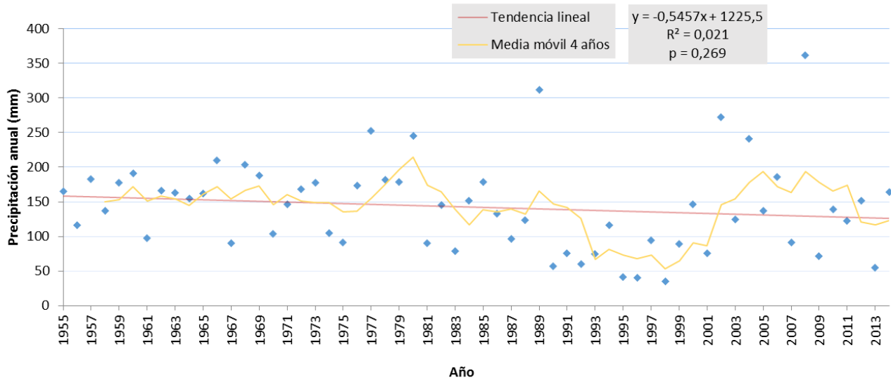
Figura 3-13. Precipitaciones anuales. Estación Meteorológica Charles Fuhr (período 1955-2014).
