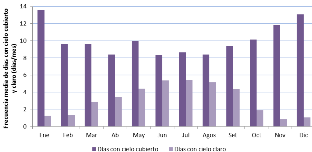
Figura 3-36. Frecuencias medias mensuales de días con cielo cubierto y con cielo claro. Estación Meteorológica Puerto Santa Cruz (período 1941-1960) y Santa Cruz Aero (período 1981-1990).
