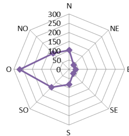
Figura 3-21. Frecuencias medias (izq.) y velocidades medias (der.) de los vientos en verano, en función de su dirección. Estación Meteorológica Puerto Santa Cruz (período 1941-1960) y Santa Cruz Aero (período 1981-1990).
