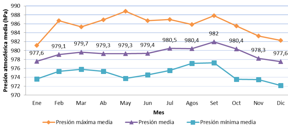
Figura 3-29. Presiones atmosféricas medias mensuales a nivel de la estación. Estación Meteorológica Lago Argentino Aero (período 1941-2000) y El Calafate (período 2001-2014). Presiones atmosféricas medias máxima y mínima mensuales a nivel de la estación. Estación Meteorológica Lago Argentino Aero (período 1981- 2000) y El Calafate (período 2001- 2010).
