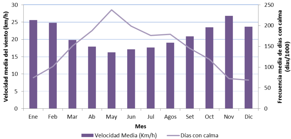
Figura 3-27. Velocidades medias mensuales del viento. Estación Meteorológica Puerto Santa Cruz (período 1941-1960) y Santa Cruz Aero (período 1981-1990).
