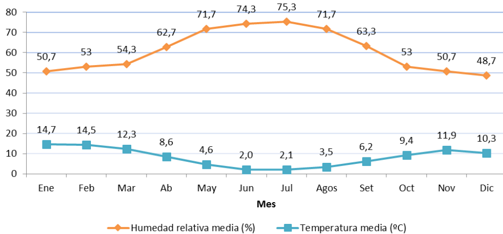
Figura 3-33. Humedad relativa media mensual. Estación Meteorológica Puerto Santa Cruz (período 1941-1960) y Santa Cruz Aero (período 1981-1990).
