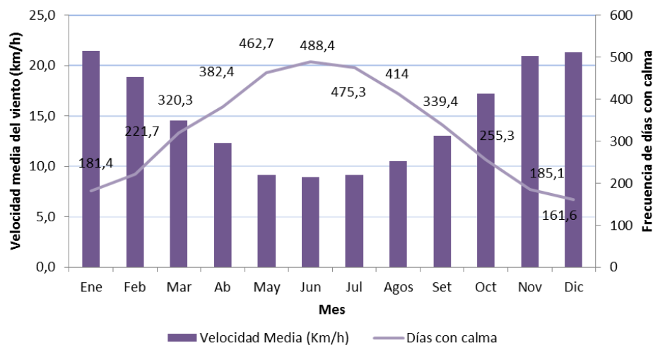
Figura 3-26. Velocidades medias mensuales del viento. Estación Meteorológica Lago Argentino Aero (período 1941-2000) y El Calafate (período 2001-2010).
