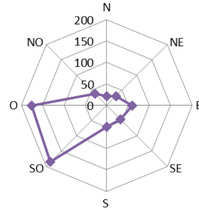
Figura 3-20. Frecuencias medias (izq.) y velocidades medias (der.) de los vientos en otoño, en función de su dirección. Estación Meteorológica Lago Argentino Aero (período 1941-2000) y El Calafate (período 2001-2010).
