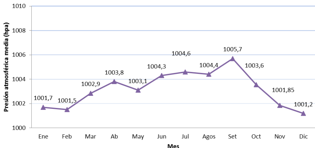
Figura 3-31. Presiones atmosféricas medias mensuales a nivel de la Estación Meteorológica Puerto Santa Cruz (período 1941-1960).
