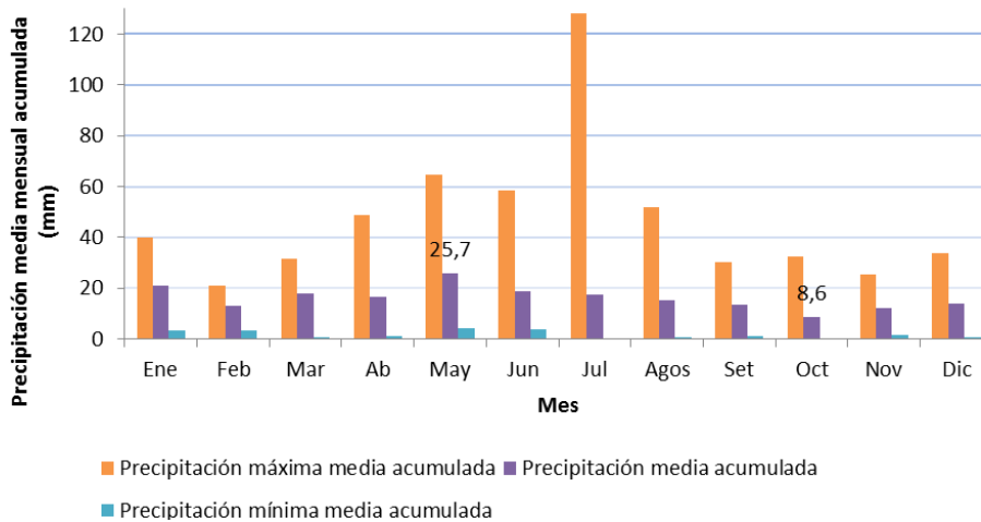
Figura 3-9. Precipitaciones medias, máximas y mínimas medias mensuales acumuladas. Estación Meteorológica Puerto Santa Cruz (período 1941-1960) y Santa Cruz Aero (período 1981-1990).
