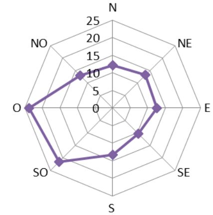
Figura 3-20. Frecuencias medias (izq.) y velocidades medias (der.) de los vientos en otoño, en función de su dirección. Estación Meteorológica Lago Argentino Aero (período 1941-2000) y El Calafate (período 2001-2010).
