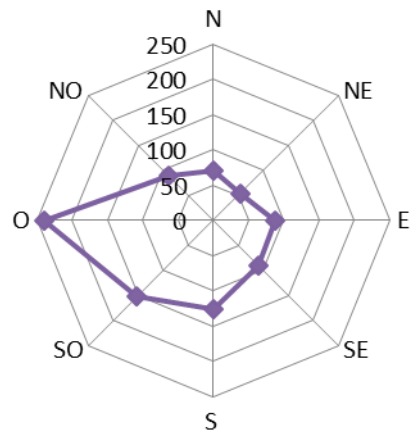
Figura 3-19. Frecuencias medias (izq.) y velocidades medias (der.) de los vientos en verano, en función de su dirección. Estación Meteorológica Puerto Santa Cruz (período 1941-1960) y Santa Cruz Aero (período 1981-1990).
