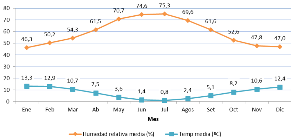
Figura 3-32. Humedad relativa media mensual. Estación Meteorológica Lago Argentino Aero (período 1941-2000) y El Calafate (período 2001-2014).
