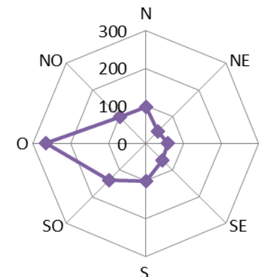
Figura 3-25. Frecuencias medias (izq.) y velocidades medias (der.) de los vientos en primavera, en función de su dirección. Estación Meteorológica Puerto Santa Cruz (período 1941-1960) y Santa Cruz Aero (período 1981-1990).
