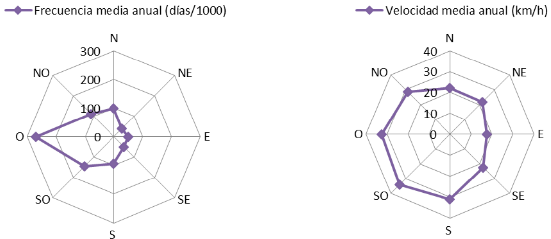
Figura 3-17. Frecuencias medias anuales (izq.) y velocidades medias anuales de los vientos (der.), en función de su dirección. Estación Meteorológica Puerto Santa Cruz (período 1941-1960) y Santa Cruz Aero (período 1981-1990).
