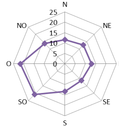
Figura 3-22. Frecuencias medias (izq.) y velocidades medias (der.) de los vientos en invierno, en función de su dirección. Estación Meteorológica Lago Argentino Aero (período 1941-2000) y El Calafate (período 2001-2010).
