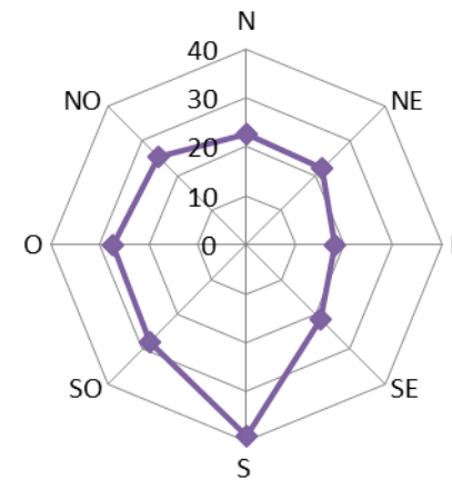
Figura 3-23. Frecuencias medias (izq.) y velocidades medias (der.) de los vientos en invierno, en función de su dirección. Estación Meteorológica Puerto Santa Cruz (período 1941-1960) y Santa Cruz Aero (período 1981-1990).
