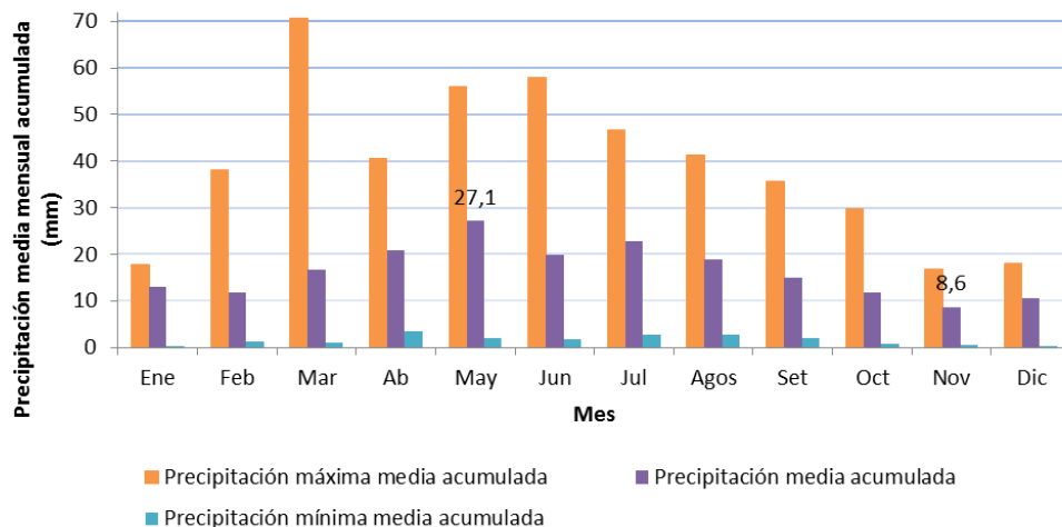
Figura 3-7. Precipitaciones medias mensuales acumuladas. Estación Meteorológica Lago Argentino Aero (período 1941-2000) y El Calafate (período 2001-2014). Precipitaciones máximas y mínimas medias mensuales acumuladas. Estación Meteorológica Lago Argentino Aero (período 1981- 2000) y El Calafate (período 2001- 2010).
