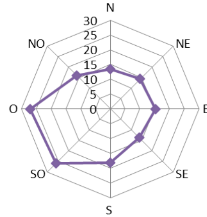
Figura 3-18. Frecuencias medias (izq.) y velocidades medias (der.) de los vientos en verano, en función de su dirección. Estación Meteorológica Lago Argentino Aero (período 1941-2000) y El Calafate (período 2001-2010).
