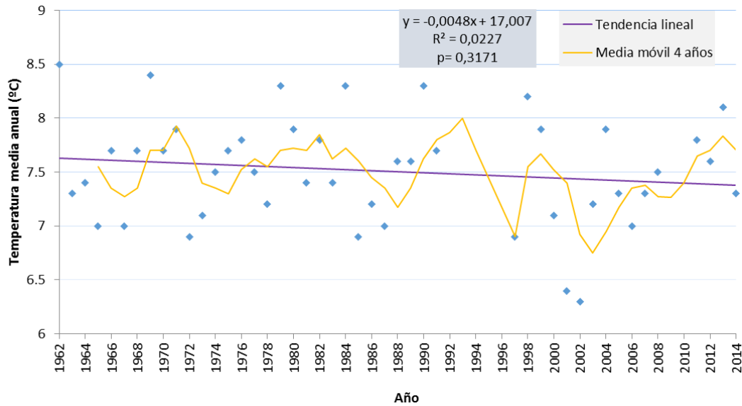
Figura 3-5. Valores medios anuales de temperatura. Estación Meteorológica Lago Argentino Aero (período 1961-2000) y El Calafate (período 2001-2014).
