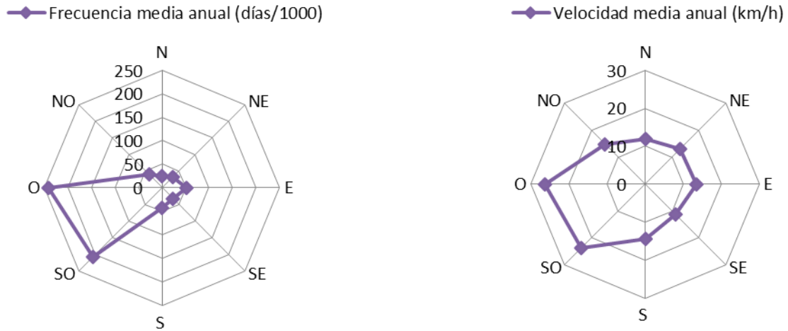
Figura 3-16. Frecuencias medias anuales (izq.) y velocidades medias anuales de los vientos (der.), en función de su dirección. Estación Meteorológica Lago Argentino Aero (período 1941-2000) y El Calafate (período 2001-2010).
