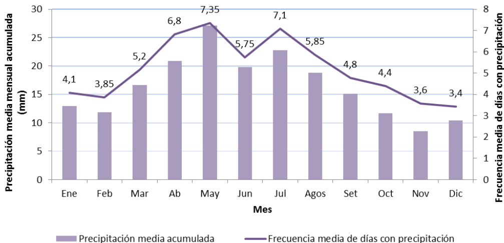
Figura 3-10. Precipitaciones medias mensuales acumuladas y frecuencias de precipitaciones medias mensuales. Estación Meteorológica Lago Argentino Aero (período 1951-2000) y El Calafate (período 2001-2010).
