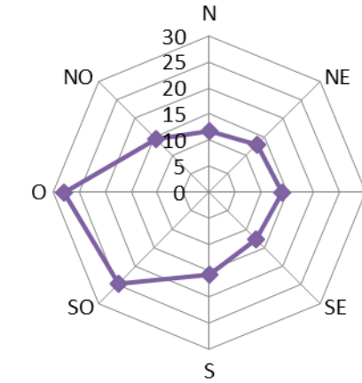
Figura 3-24. Frecuencias medias (izq.) y velocidades medias (der.) de los vientos en primavera, en función de su dirección. Estación Meteorológica Lago Argentino Aero (período 1941-2000) y El Calafate (período 2001-2010).
