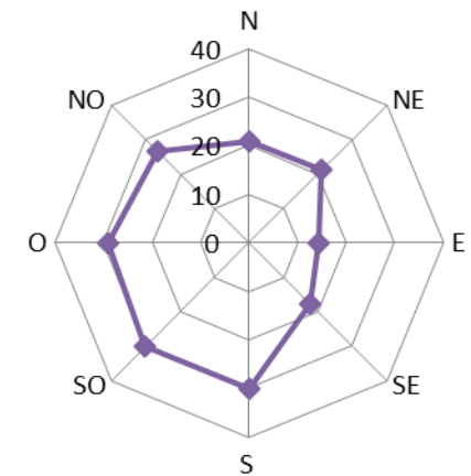
Figura 3-21. Frecuencias medias (izq.) y velocidades medias (der.) de los vientos en verano, en función de su dirección. Estación Meteorológica Puerto Santa Cruz (período 1941-1960) y Santa Cruz Aero (período 1981-1990).
