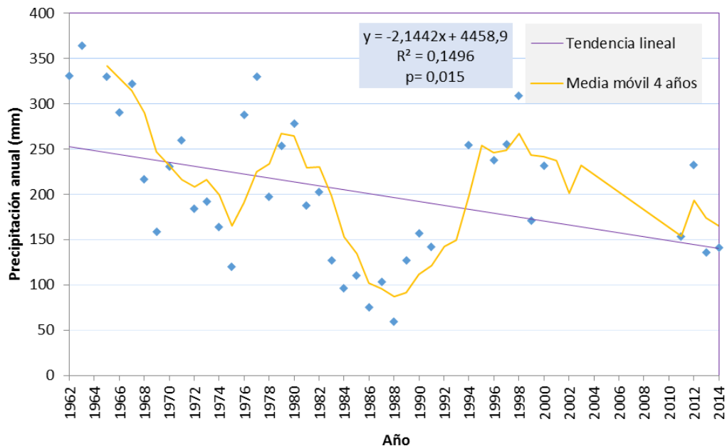
Figura 3-12. Precipitaciones anuales. Estación Meteorológica Lago Argentino Aero (período 1961-2000) y El Calafate (período 2001-2014).
