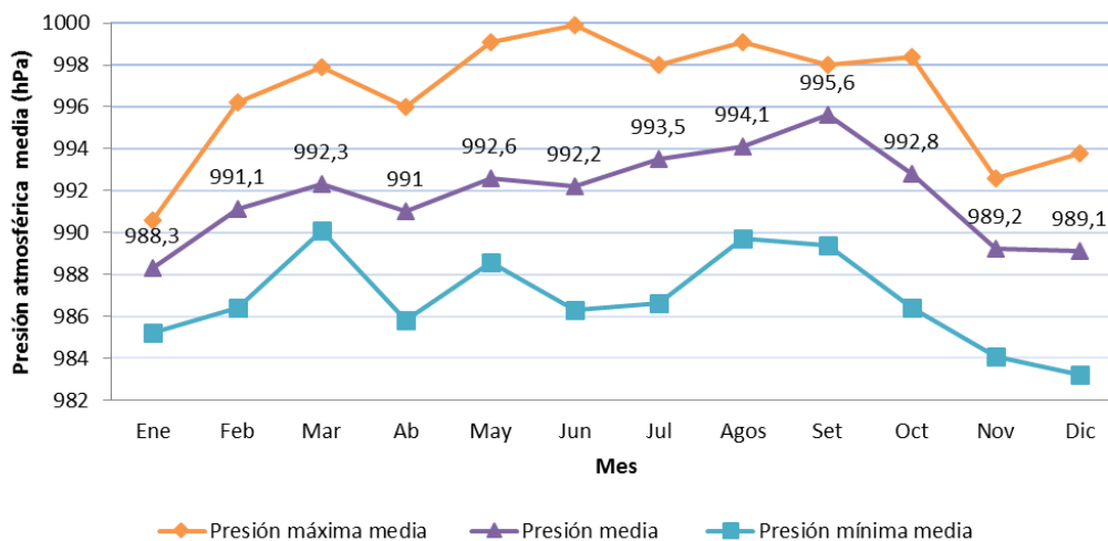
Figura 3-30. Presiones atmosféricas medias, máximas y mínimas medias mensuales a nivel de la estación. Estación Meteorológica Santa Cruz Aero (período 1981-1990).
